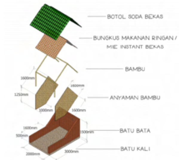
Gambar 4.22 — Ilustrasi aksonometri kios Pasar Cendani
