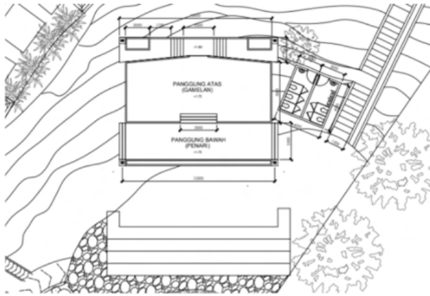
Gambar 4.9 — Desain layout panggung gamelan Begaganlimo
