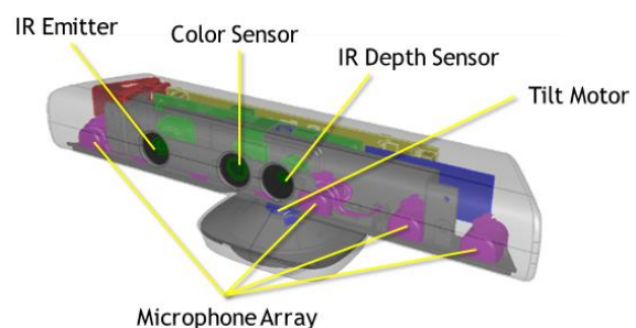
Gambar 1. Sensor-sensor pada perangkat Kinect (Microsoft Library)
