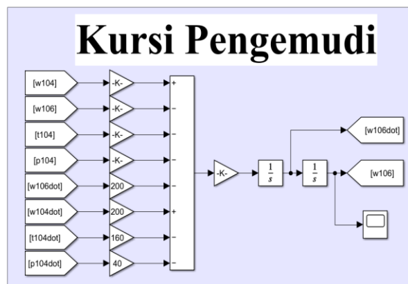
Gambar 7. Block Simulink tempat duduk truk
