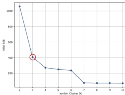
Gambar 2. Plot Elbow Berdasarkan Data LRFM Pelanggan
