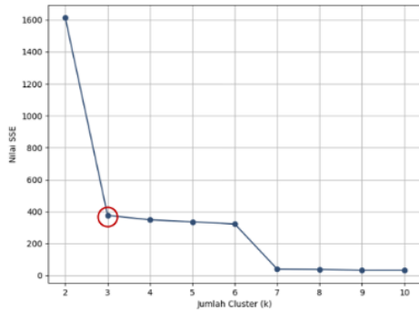
Gambar 3. Plot Elbow Berdasarkan Data MLRFM Pelanggan
