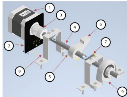
Gambar 5. Bagian Penggeser Otomatis
