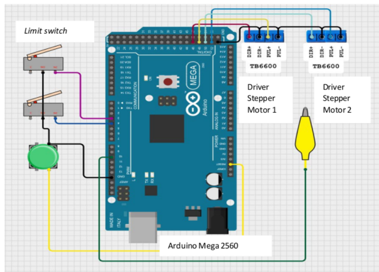
Gambar 8. Wiring Diagram untuk Sistem Pengarah Otomatis
