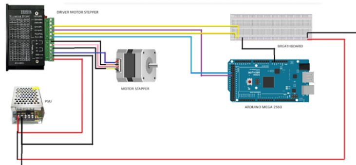
Gambar 7. Wiring Diagram untuk Sistem Penarik Strip
