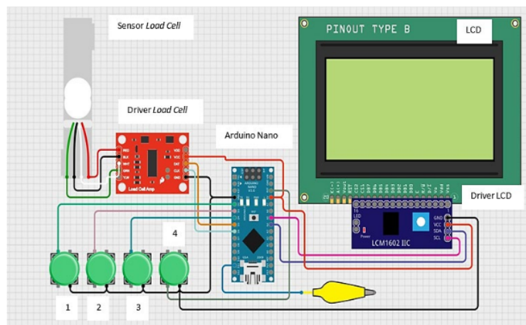
Gambar 9. Wiring Diagram untuk Sistem Penggulung, Load Cell, Layar dan Tombol
