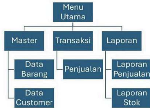
Gambar 5. Desain menu program aplikasi penjualan dan persediaan
