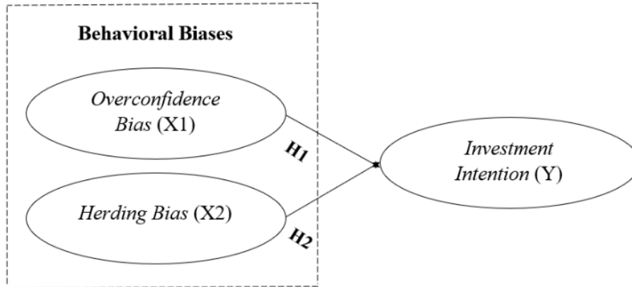
Gambar 1. Kerangka Penelitian
