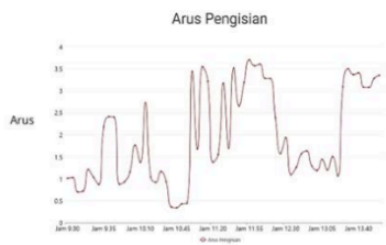
Gambar 15. Grafik arus pengisian 30 Desember 2022
