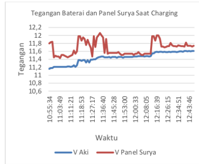
Gambar 12. Grafik Tegangan pada Baterai dan Panel Surya 21 November 2022
