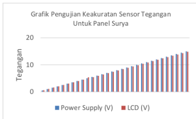
Gambar 11. Grafik Pengujian Keakuratan Sensor Tegangan Untuk Panel Surya
