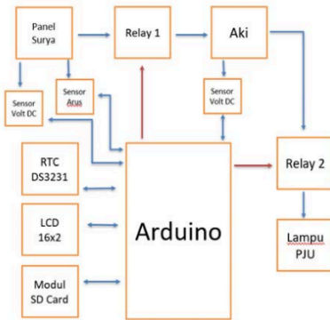
Gambar 6. Diagram Perancangan Sistem
