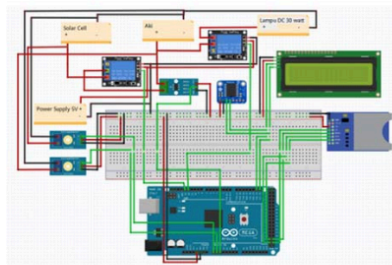
Gambar 9. Rangkaian Keseluruhan Sistem
