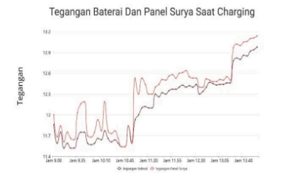
Gambar 13. Grafik Tegangan pada Baterai dan Panel Surya 30 Desember 2022
