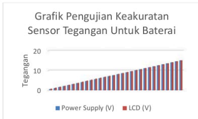
Gambar 10. Grafik Pengujian Keakuratan Sensor Tegangan Untuk Baterai
