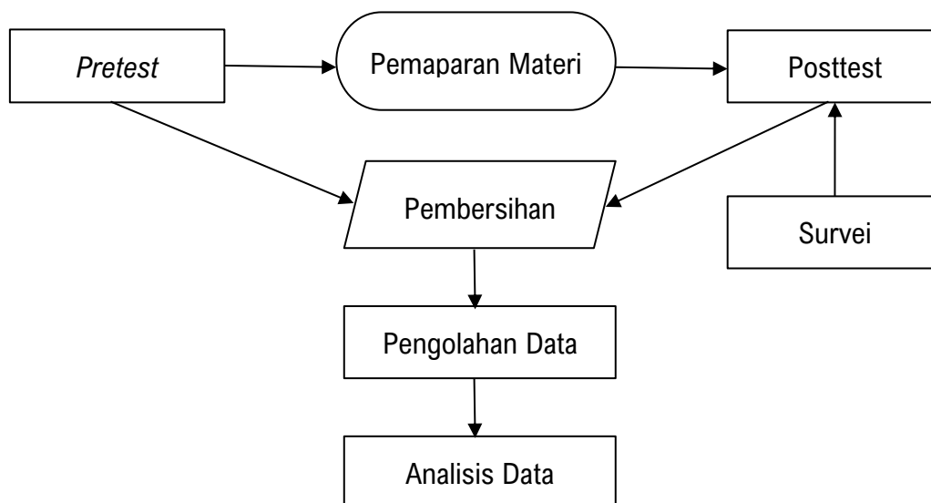
Gambar 1. Desain Penelitian
